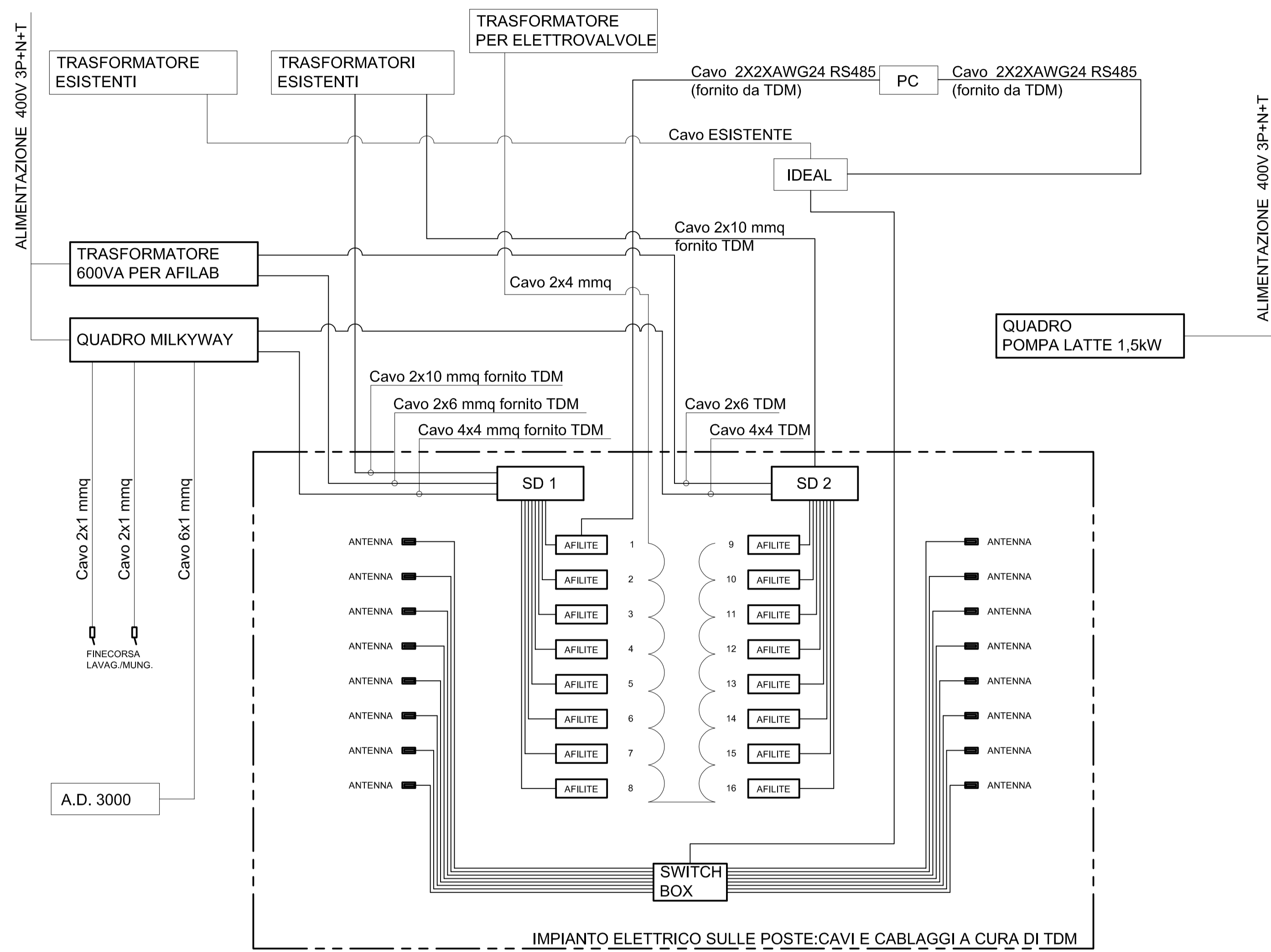
IMPIANTO ELETTRICO SULLE POSTE: CAVI E CABLAGGI A CURA DI TDM
